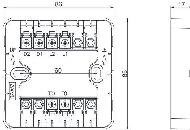
Figure2 JK-A52E Module Base(DZ-A52)
